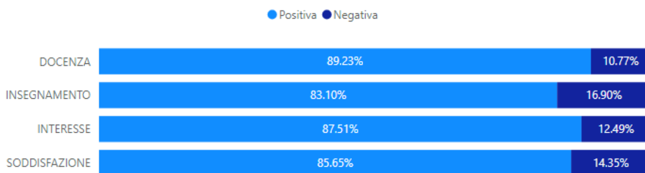
Figura 1. Valutazione dei questionari per macrosezioni.
